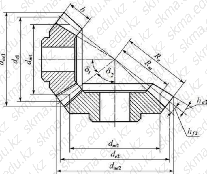
5-сурет. Конусты тісті берілістің геометриялық параметрлері
