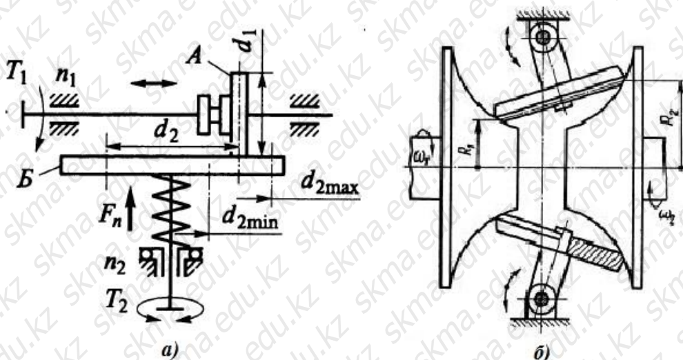
21-сурет. Вариаторлар
