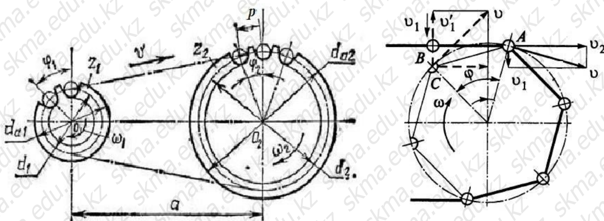
17-сурет. Шынжырлы берілістердің геометриясы мен кинематикасы
