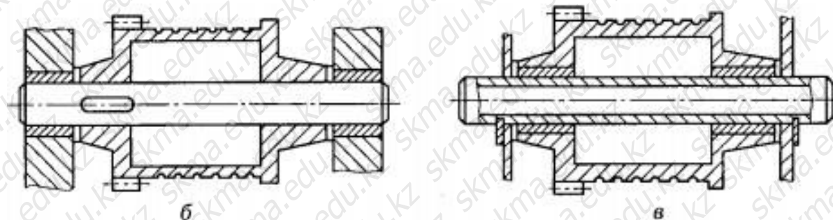
30-сурет. Қозғалмайтын және айналмалы осьтер конструкциясы
